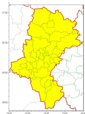
Opady marznące 2021-01-19 12:16
